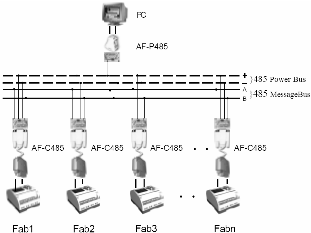
Рис. 2.12 Способ подключения
