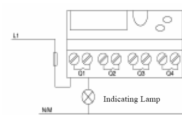
Рис. 2.10 Релейный выход
