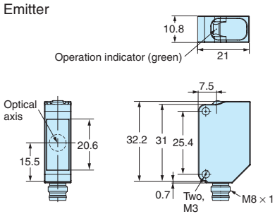
Emitter
