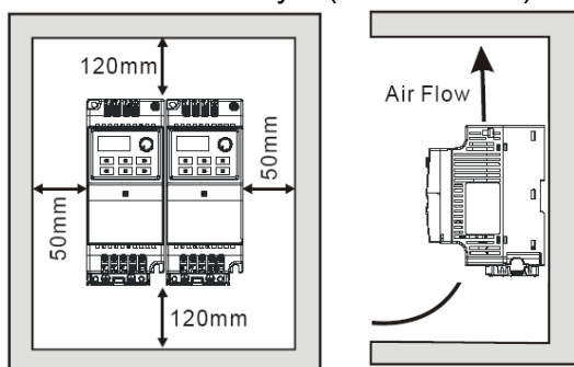
Установка вплотную (-10 ... +40°C)
