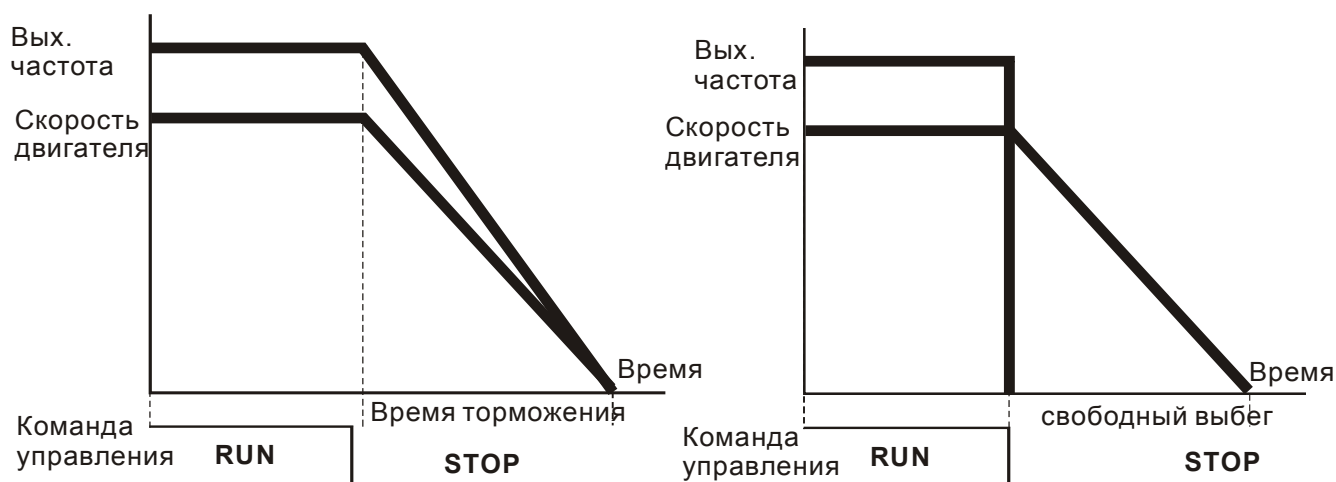
Остановка с замедлением и на выбеге
