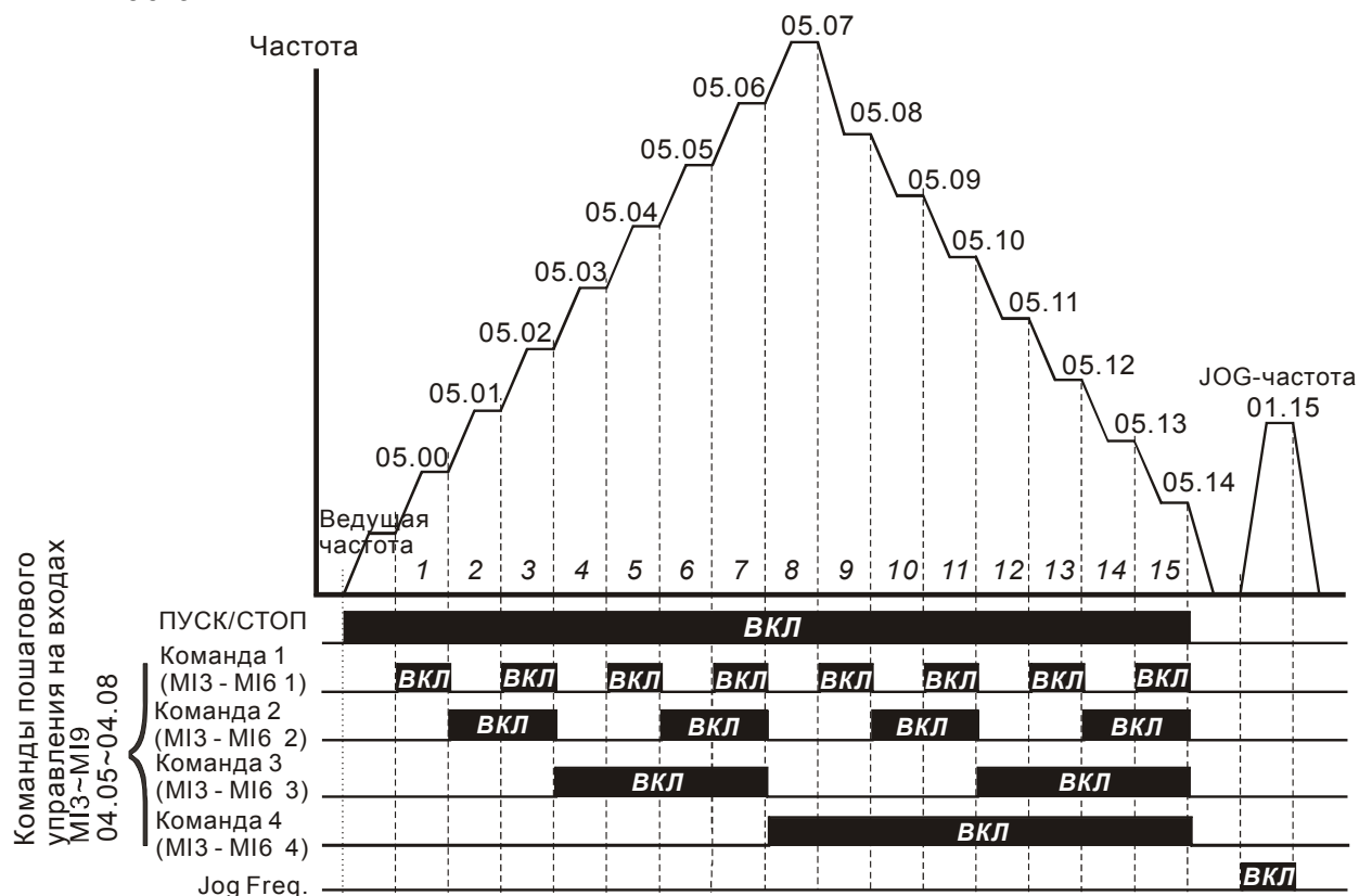
Пошаговое управление скоростью через внешние терминалы
