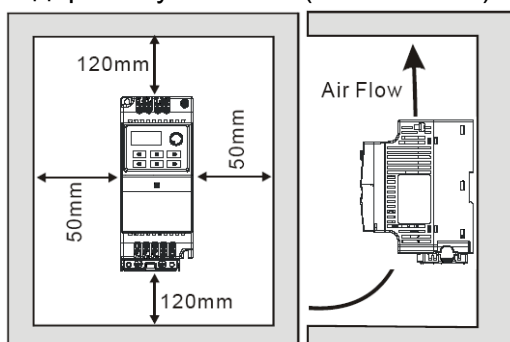
Стандартная установка (-10 ... +50°C)
