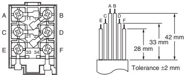
(2 conduits type)
