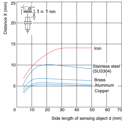
E2E2-X14MD□
