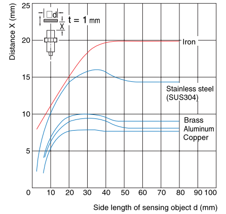
E2E2-X20MD□
